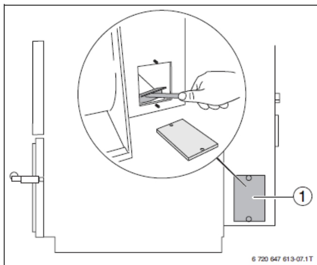
Фиг. 27 Страничен отвор за почистване на колектора за димни газове
